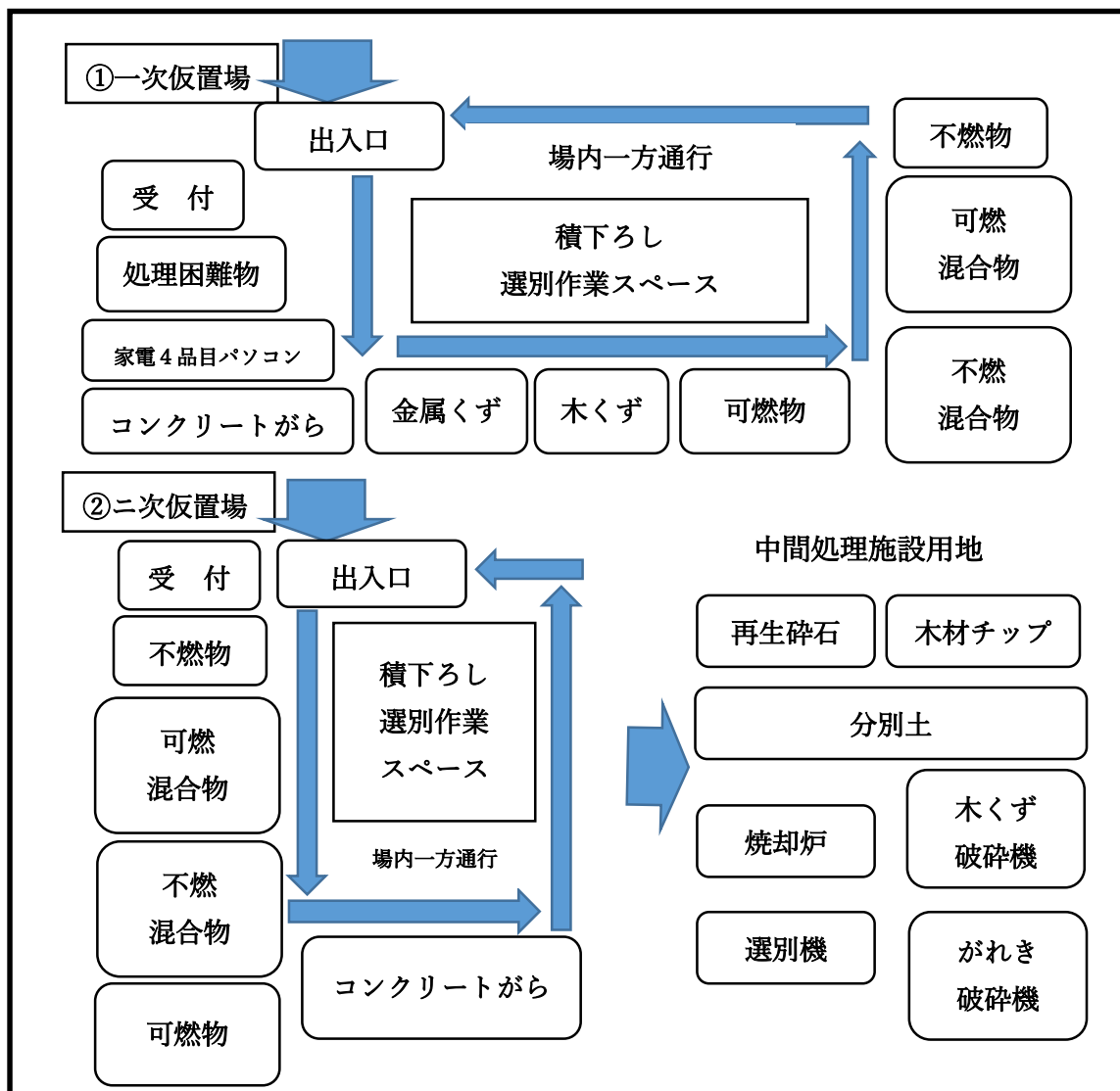
図3-4 仮置場のレイアウト例
