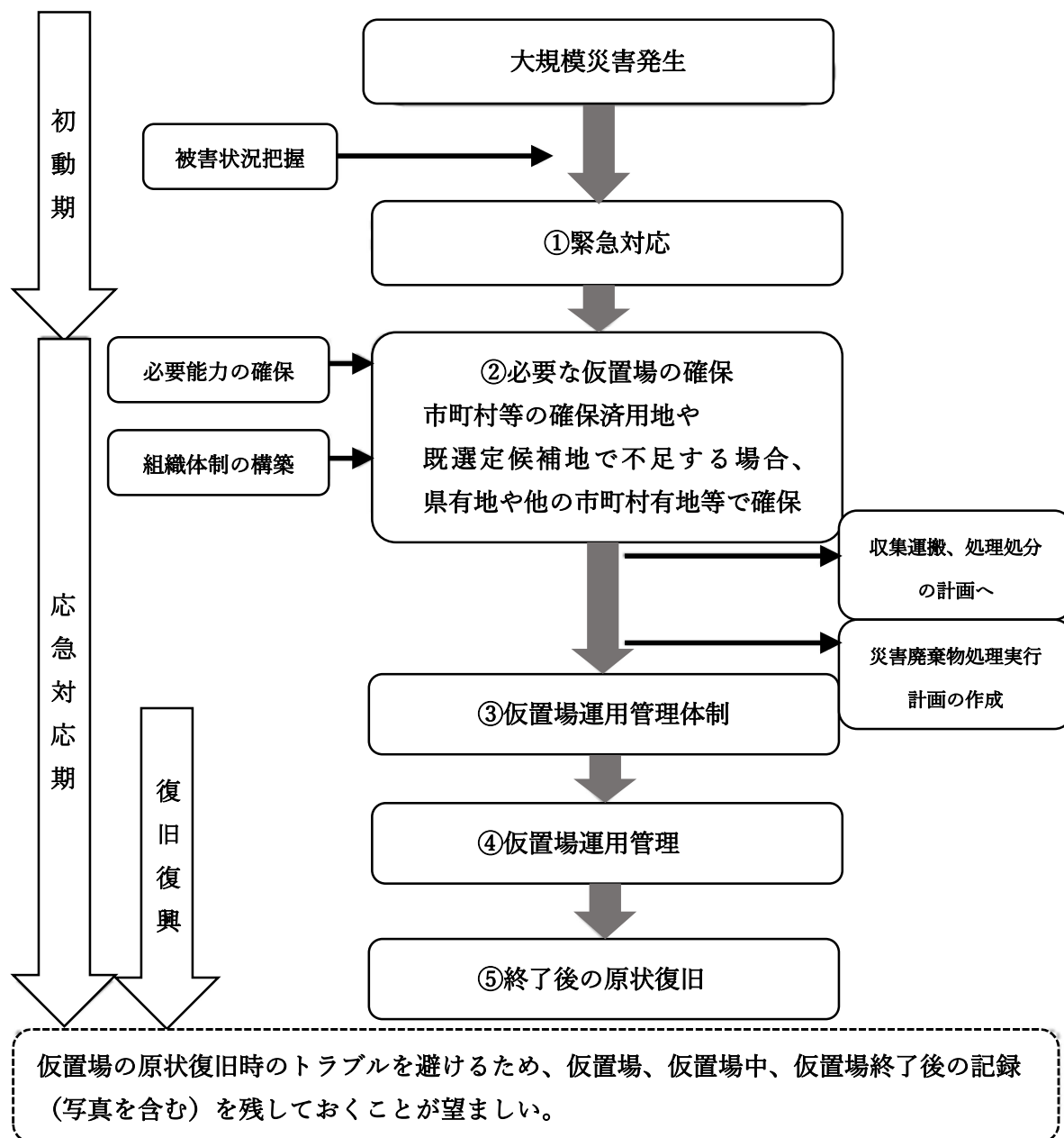
図3-3 仮置場の確保及び運営管理に係るフロー
